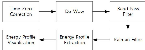
그림 2. GPR 신호처리 절차
