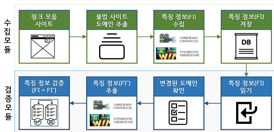
그림 5. 특징 정보 수집 및 검증 과정 Fig. 5. Process of Collecting and Verifying Feature Information
