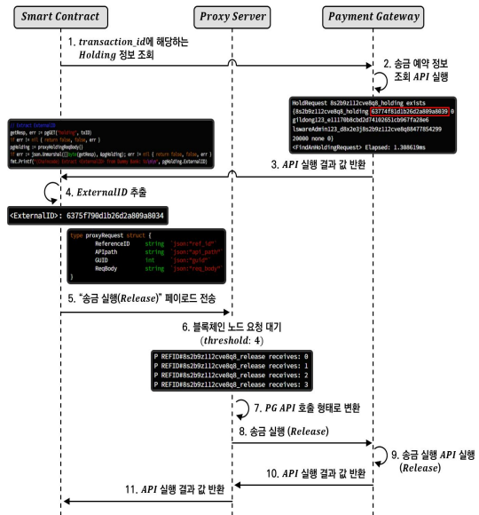
그림 6. 송금 실행(Release) 시퀀스 Fig. 6. Transfer Release Sequence
