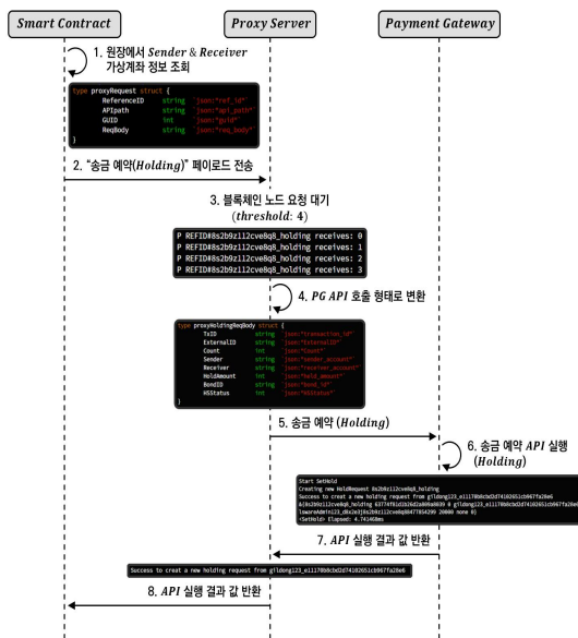
그림 5. 송금 예약(Holding) 시퀀스 Fig. 5. Transfer Holding Sequence
