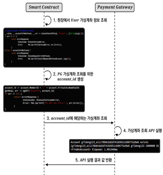
그림 4. PG 가상계좌 정보 조회 시퀀스 Fig. 4. PG Virtual Account Query Sequence
