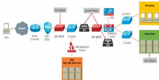
그림 1. 컴퓨팅 시스템 보안 계층 구조 Fig. 1. Computing System Security Hierarchy
