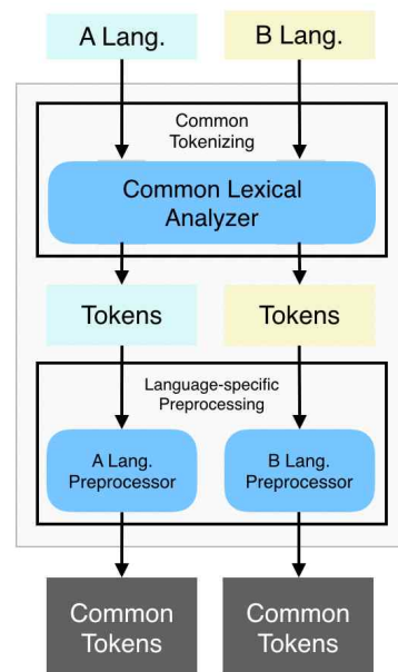
그림 2. 공통 토큰 생성 방법 Fig 2. Method for Common Token Generation
