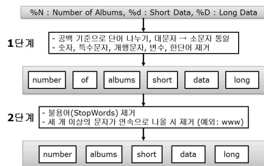
그림 2. 문자열 정제 절차
