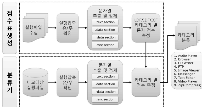
그림 1. 문자열 정보를 이용한 소프트웨어 분류 기법 개요
