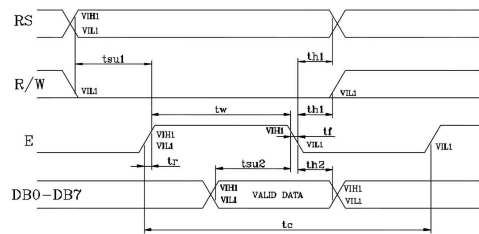
그림 3. LCD timing diagram
